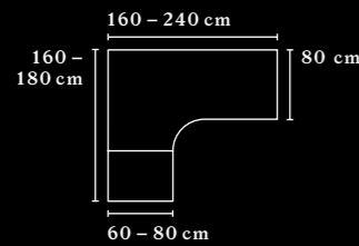
KOMBITISCH K3 COMBINATION DESK K3
