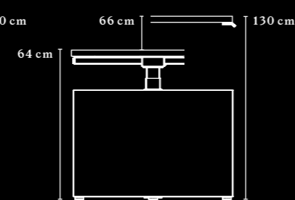
3-teilige Säule, elektrisch höhenverstellbar Three-part column, electrically height adjustable
