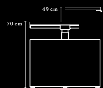
2-teilige Säule, elektrisch höhenverstellbar Two-part column, electrically height adjustable
