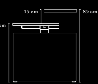
Höheneinstellbar 20-mm-Raster mit Werkzeug Height adjustable in 20 mm grid with tool
