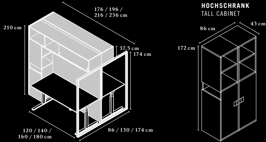
2 ARBEITSPLÄTZE 2 WORKSTATIONS
